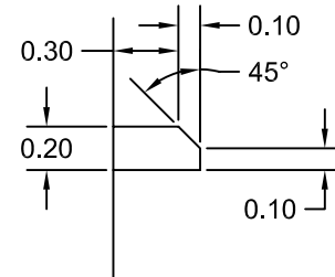
DETAIL: A SCALE : 2x
